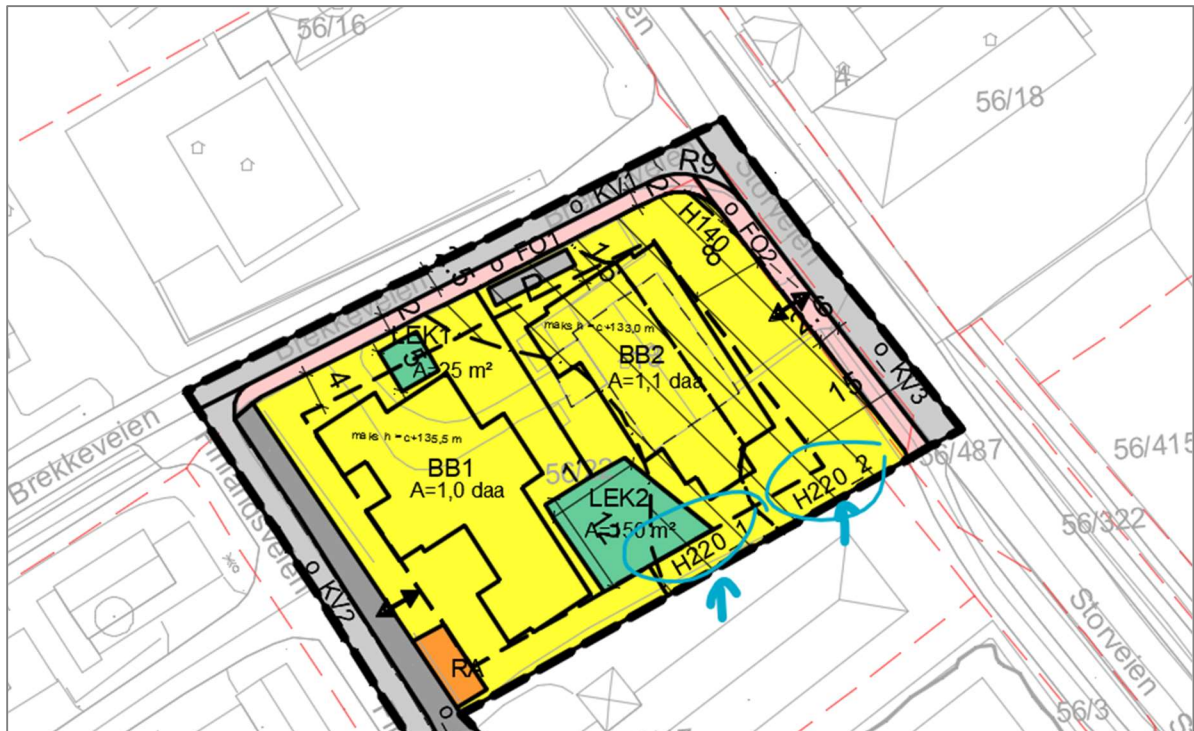
Plankartet viser endring i støyforhold etter utbygging av trinn 2 sammenlignet med trinn 1
