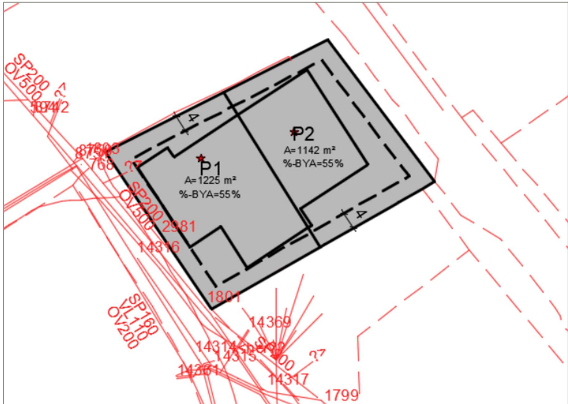
Utsnitt som viser plannivå 1 sammen med eksisterende ledningsnett.
